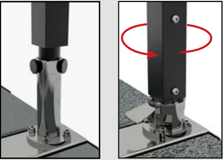
Standardfuß für die Amalfi-Masten Typ S und N Pied standard pour les mâts Amalfi Type S et N
